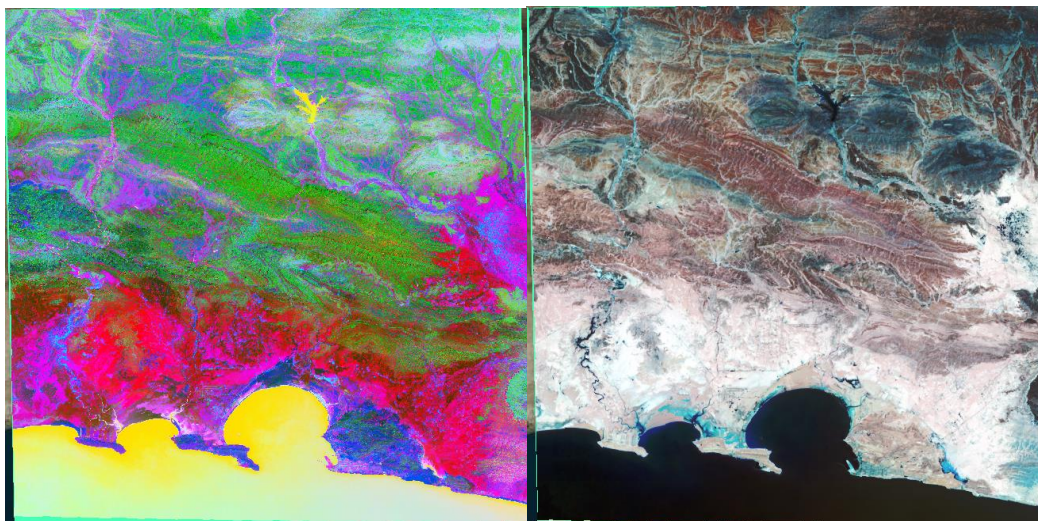
شکل ۳-۱۴- سمت راست) تصویر یکپارچه شده سنجنده MSI مربوط به Sentinel-2 از ناحیه مورد مطالعه (ترکیب باندی ۲-۴-۹). سمت چپ) نمایش مؤلفه‌های ۱، ۳ و ۴ تحلیل مؤلفه‌های اصلی (PCA) تصویر Sentinel-2 مرتبط با ناحیه مورد مطالعه.
