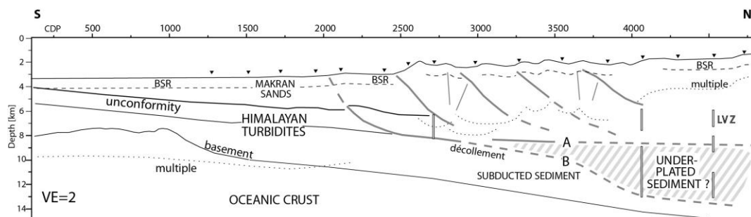
شکل ۵-۲- ساختار گوه افزایشی مکران، نشان‌دهنده رسوبات زیرصفحه‌ای در زیر یک دکلومان با شیب ملایم (Kopp et al., 2000).
