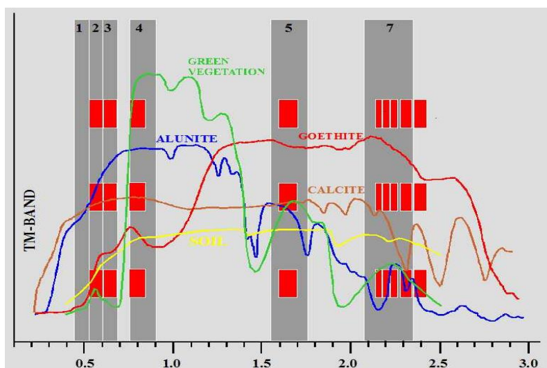
شکل ۳-۲- مقایسه قدرت تفکیک طیفی تصاویر ETM و ASTER
