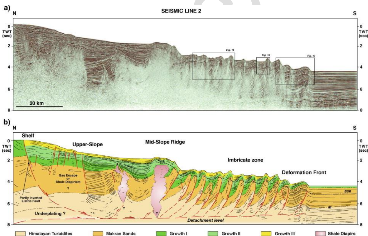
شکل ۶-۲- برش لرزه‌ای (a) و تفسیر (b) در امتداد گوه افزایشی مکران در فراساحل باختری، نشان‌دهنده فلات قاره‌ای، حوضه‌های شیبی و منشور افزایشی. ناپوستگی M توربیدیت‌های هیمالیایی را از ماسه‌سنگ‌های مکران جدا می‌کند. تفسیر نشان‌دهنده لایه‌های رشد، دیابیرهای شیلی، منطقه به-هم‌پیوسته و جبهه دگرشکلی است، همچنین پتانسیل زیرصفحه‌ای و یک سطح جدایش را شناسایی کرده است (Grando and McClay, 2007).
