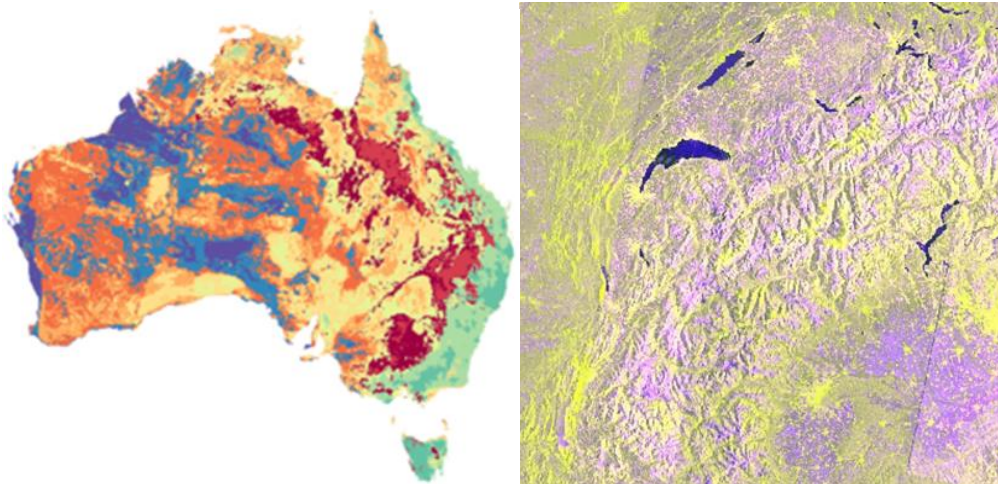
شکل ۳-۸- تصویر سمت راست) نمایی از تصویر Sentinel-1 SAR GRD. تصویر سمت چپ) ویژگی‌های خاک در گستره استرالیا با استفاده از داده‌های Soil and Landscape Grid (SLGA).
