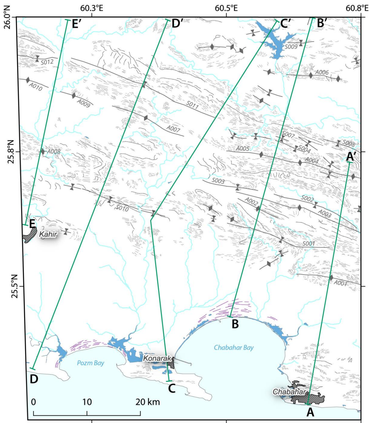
شکل ۵-۱- نقشه چین‌خوردگی که تاقدیس‌ها و ناودیس‌های موجود در منطقه مورد بررسی SUTGMM را نشان می‌دهد. خطوط سبز (AA' تا EE') نمایانگر خطوط برش‌های عرضی هستند که برای ساخت برش‌های ترازمند استفاده شده‌اند.
