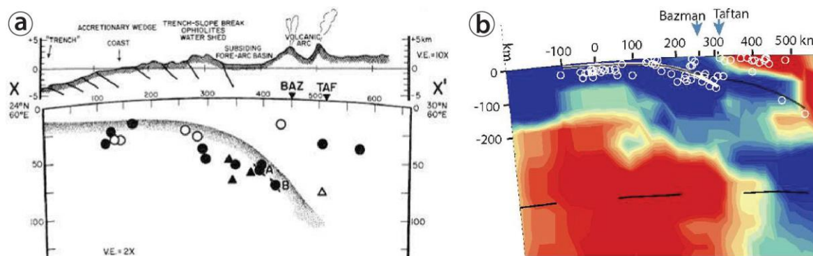
شکل ۲-۴- (a) برش شمالی-جنوبی در مکران باختری ( 60^{\circ}\text{E} ) که فرورانش صفحه عربی به زیر صفحه اوراسیا را نشان می‌دهد، همراه با رویدادهای لرزه‌ای که در امتداد این برش تصویر شده‌اند و نشان‌دهنده افزایش شیب فرورانش زیر فرونشست جازموریان است (Jacob et al., 1979). (b) توپوگرافی لرزه‌ای (Hafkenscheid et al., 2006) و زمین‌لرزه‌ها با صفحه فرورونده در زیر منطقه مکران (Dolati, 2010).
