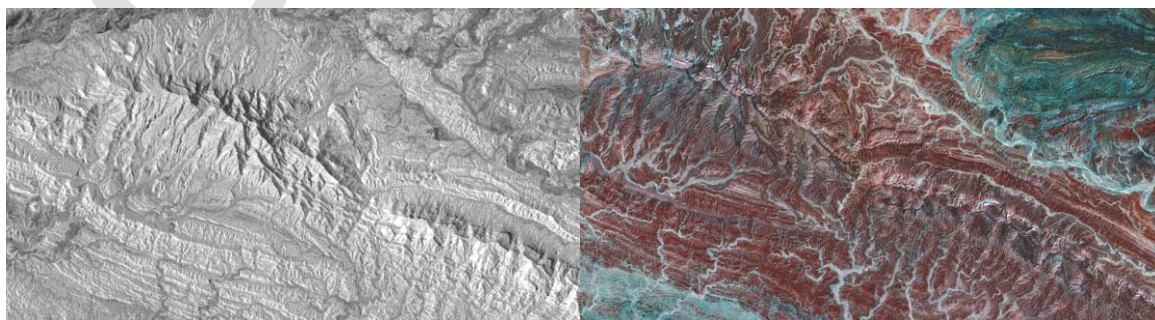
شکل ۳-۱۵- سمت راست) تصویر یکپارچه شده سنجنده MSI مربوط به Sentinel-2 از ناحیه مورد مطالعه (ترکیب باندی ۲-۴-۹). سمت چپ) تصویر Sentinel-1 با باند VH از ناحیه مورد مطالعه.
