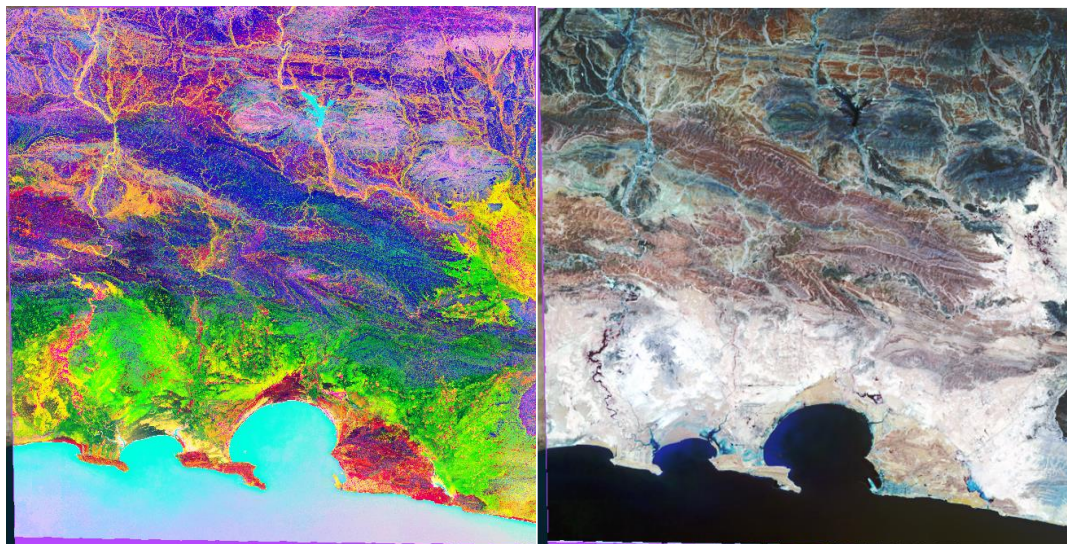
شکل ۳-۱۳- سمت راست) تصویر یکپارچه شده سنجنده LOI مربوط به لندست ۸ مرتبط با محدوده مطالعاتی (ترکیب باندی ۲-۴-۶). سمت چپ) نمایش مؤلفه‌های ۱، ۲ و ۳ تحلیل مؤلفه‌های اصلی (PCA) تصویر لندست ۸ مرتبط با محدوده مطالعاتی.
