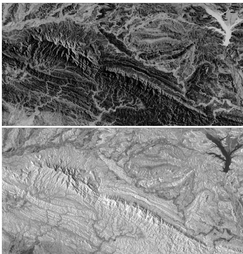
شکل ۳-۱۶- نمایشی نزدیک از تصویر راداری بخش خاوری محدوده مطالعاتی. تصویر بالایی و پایینی به ترتیب برداشت VV و VH می‌باشند.
