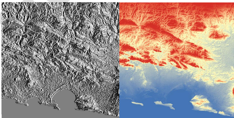
شکل ۳-۱۷- راست) تصویر مدل رقومی ارتفاع سنجنده SRTM محدوده مطالعاتی. چپ) تصویر Hillshade از ناحیه مورد مطالعه.
