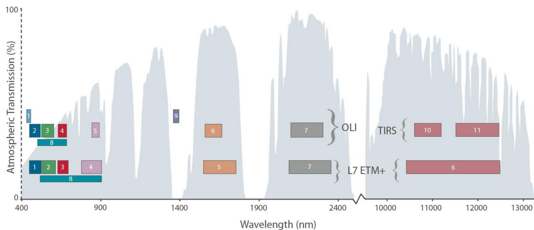
شکل ۱-۳- مقایسه پهنای باندهای لندست ۷ با لندست ۸ و موقعیت هر کدام از آنها نسبت به پنجره‌های اتمسفری (منبع:
