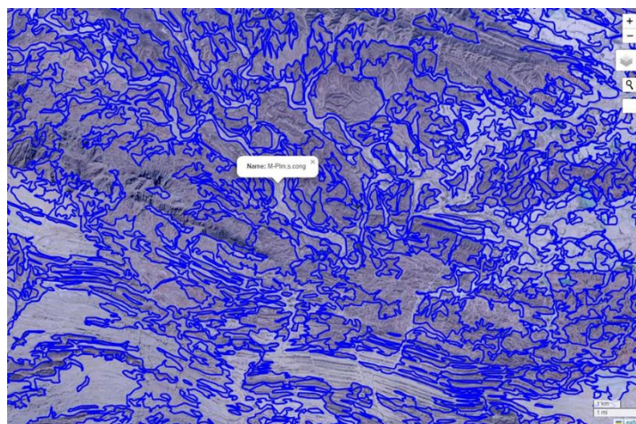
شکل ۳-۴۰- لایه زمین‌شناسی تولید شده با قابلیت جستجوی ویژگی‌های هر واحد.
