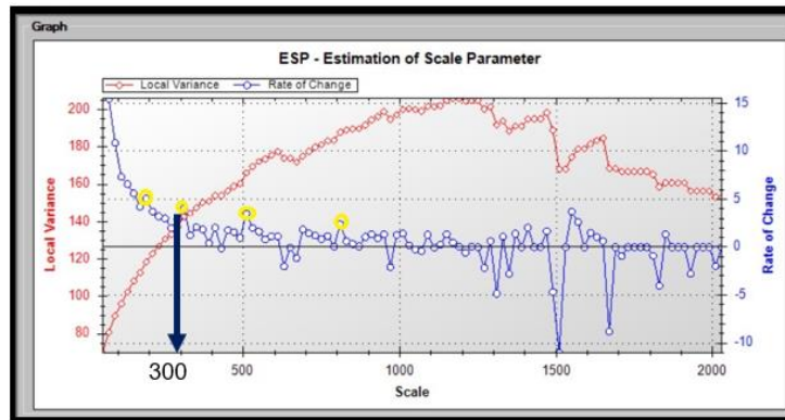
شکل ۳-۲۰- تغییرات واریانس محلی و دامنه تغییر در مقیاس‌های مختلف.
